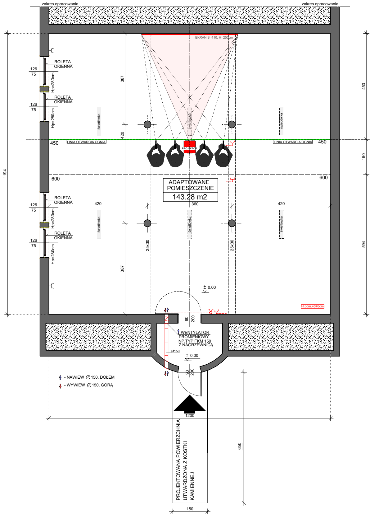
RZUT PRZYZIEMIA - ADAPTACJA POMIESZCZENIA W ZESPOLE SZKÓŁ ZAWODOWYCH im. PIASTÓW OP. W KRAPKOWICACH NA POTRZEBY UTWORZENIA WIRTUALNEJ STRZELNICY.
